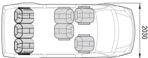
ГАЗ - 22171 «СОБОЛЬ»
