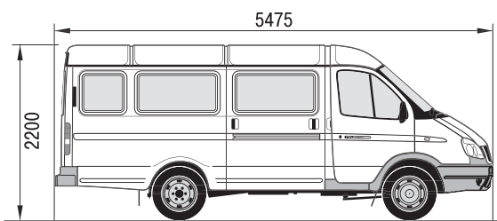
ГАЗ - 3221 «ГАЗЕЛЬ»
