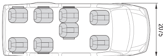
ГАЗ - 3221 «ГАЗЕЛЬ»
